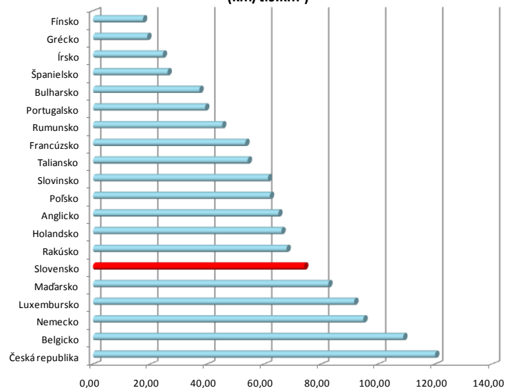
Hustota železničnej siete vo vybraných krajinách Európy (km/tis.km 2 )
